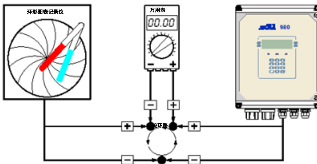
图 29 从环路断开 4 - 20mA 设备进行校准
