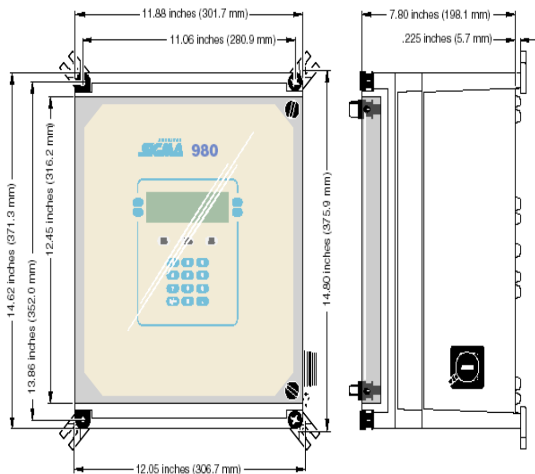
图 5 安装尺寸 (1)
