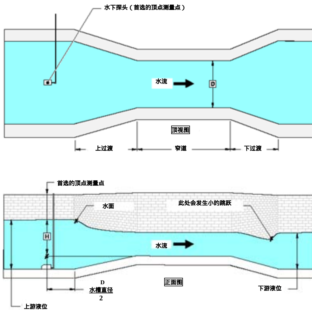
图 52 Palmer-Bowlus 型水槽
