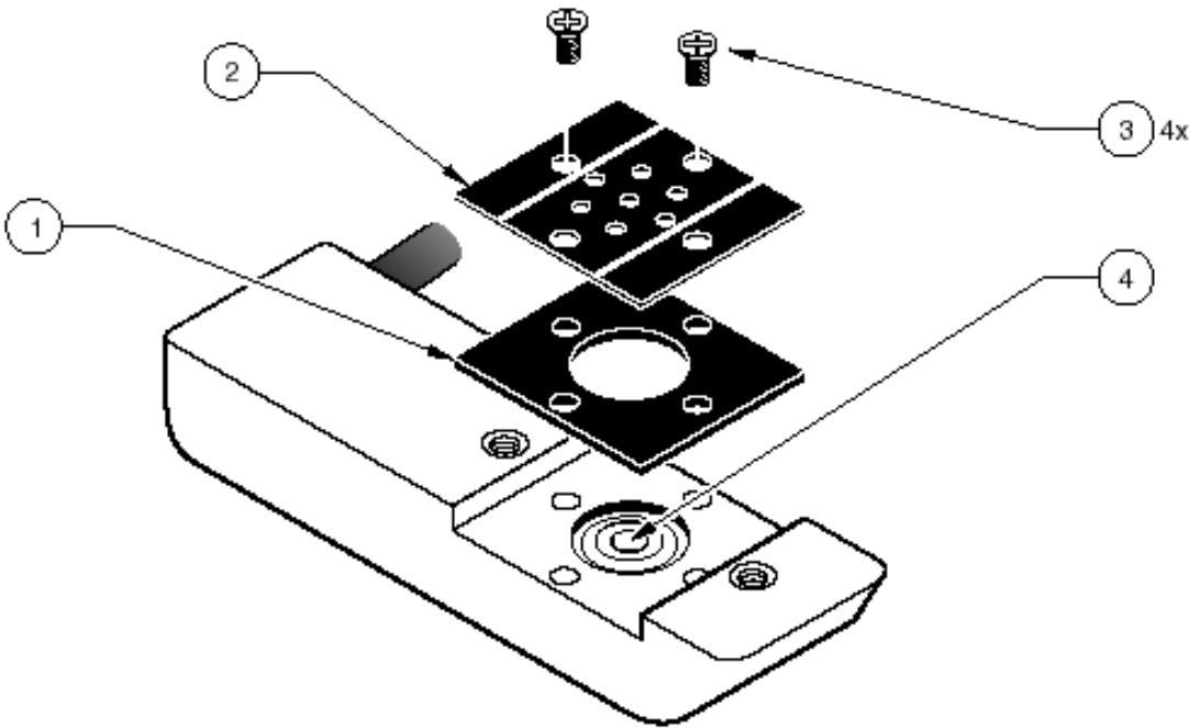
图 47 移开保护盖
