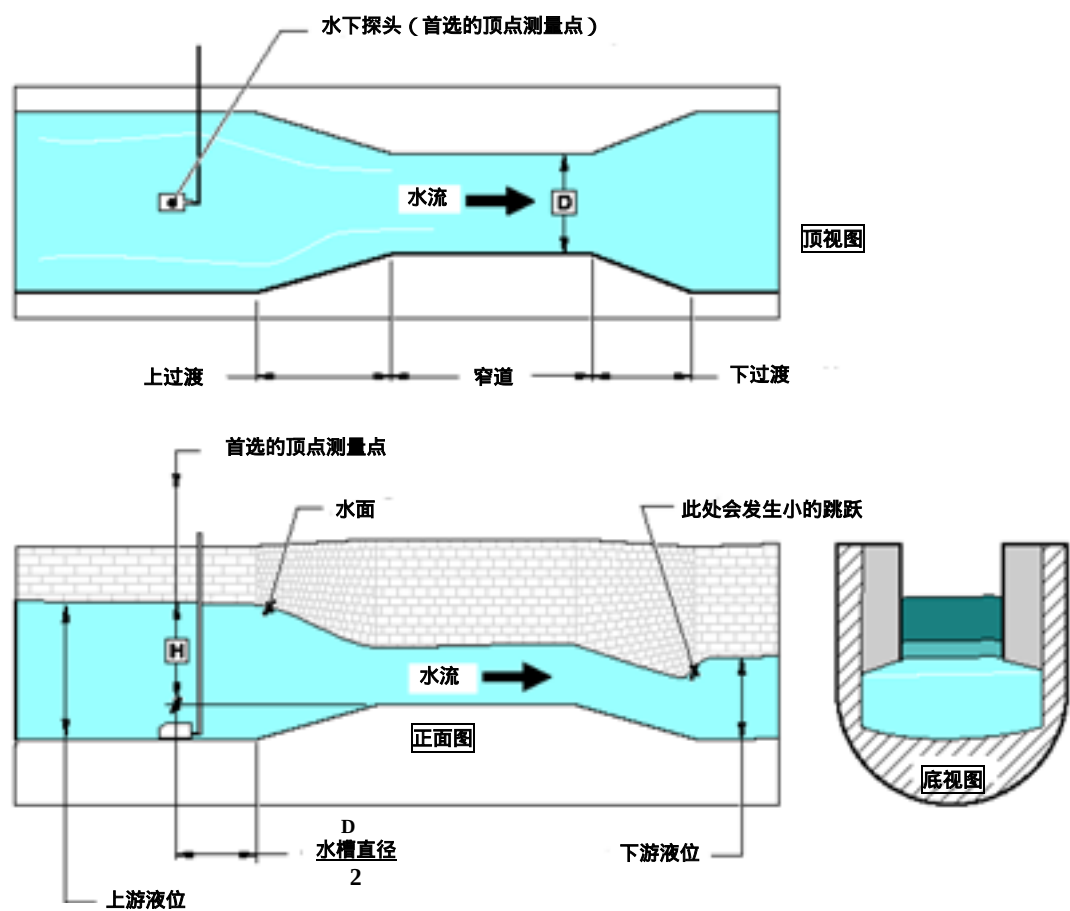
图 53 Leopold-Lagco 型水槽
